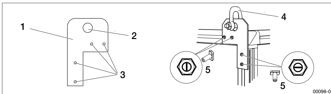
Joonis: Tõstekronstein EMMT-12
