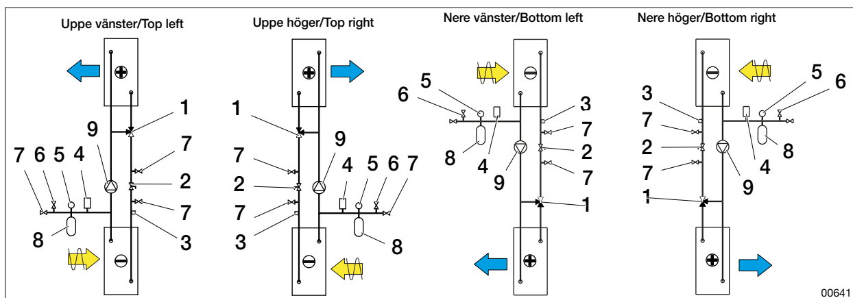
Afbeelding: Schematische weergave terugwinningscircuit
