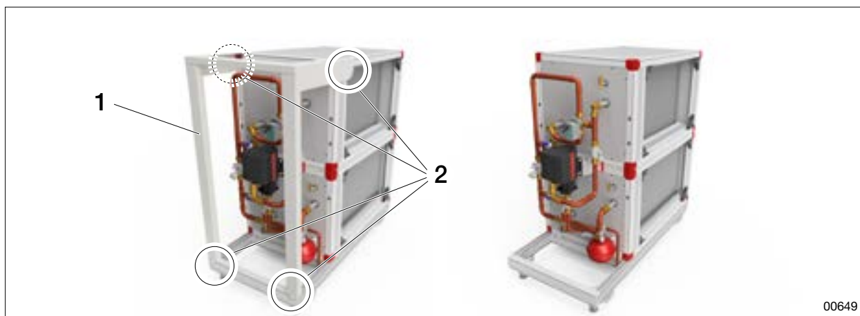
Afbeelding: Transportbescherming
